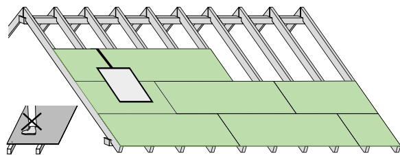
Verlegeprinzip Unterdeckung (schematische Darstellung). Platten nur im Sparrenbereich begehen. Verlegehinweise in der Broschüre Dach-Technik.
