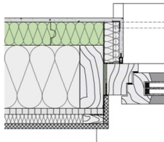
Einsatz im WDVS-System
